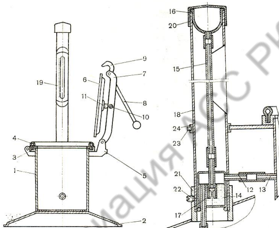
Рис.133. Схема прибора ПГС
