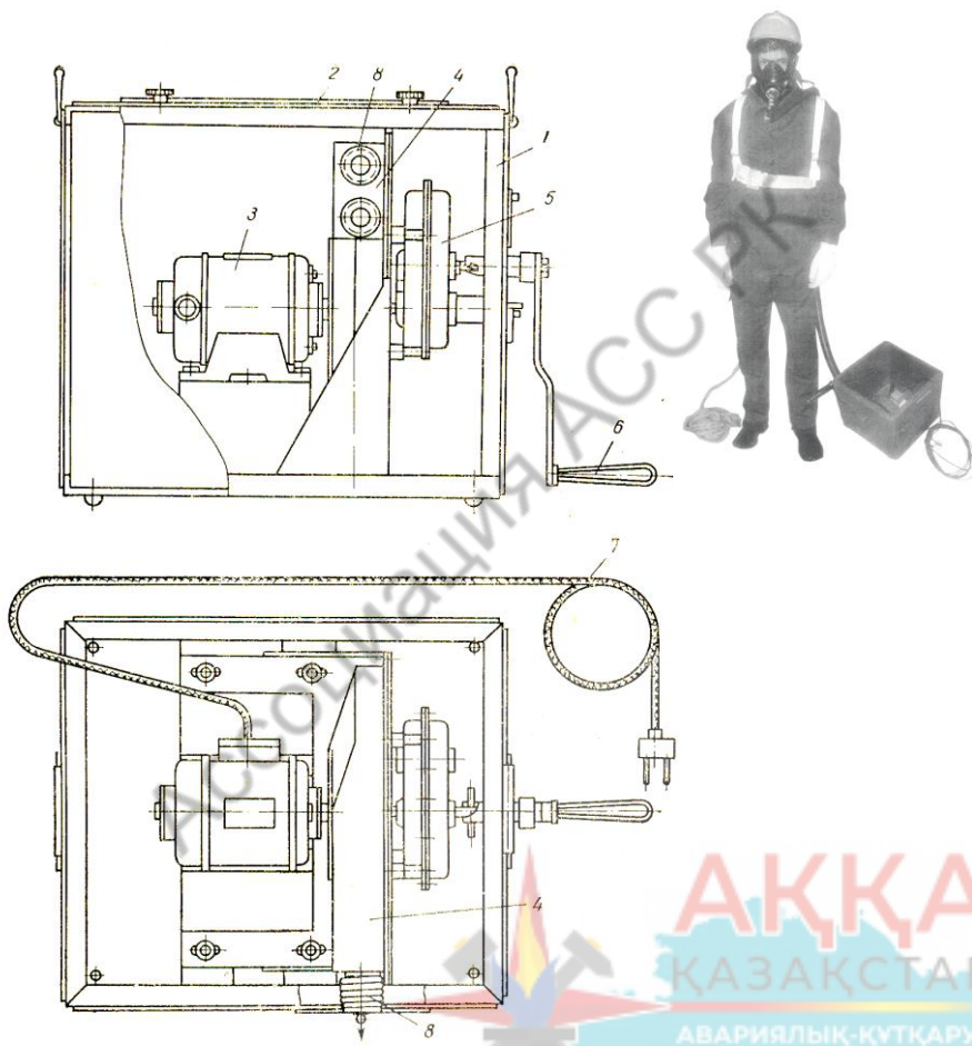
Рис. 12. Электровоздуходувка для противогаза типа ПШ-20:
