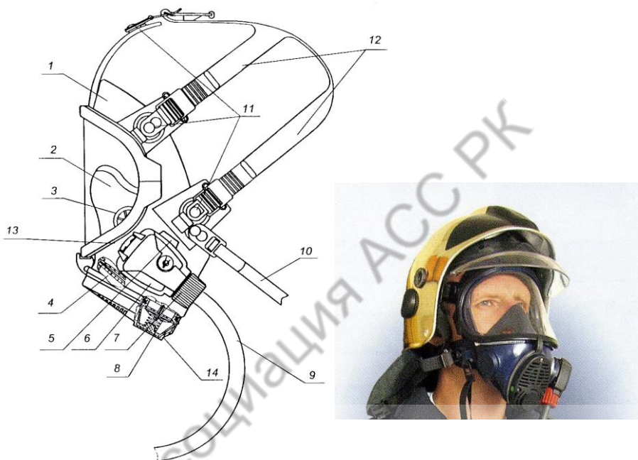
Рис. 29. Маска «Пана Сил» из неопрена или силикона с резиновым или сетчатым оголовьем с легочным автоматом (вариант 2)
