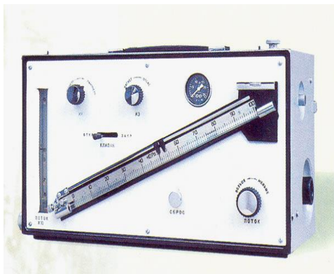
Рис. 127. Контрольный прибор УКП-5
