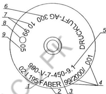
Рис. 20. Маркировка стального баллона фирмы «FABER»
