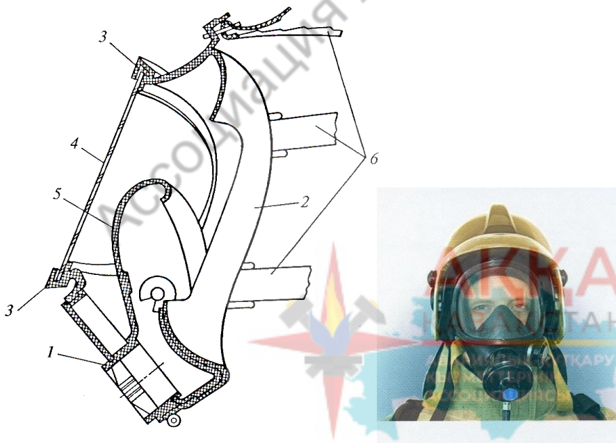
Рис. 25. Панорамная дыхательная маска ПМ-88М
