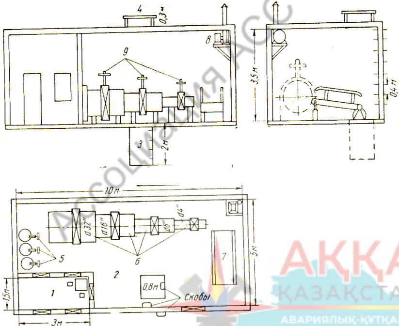
Рис.1. Газодымная камера:
