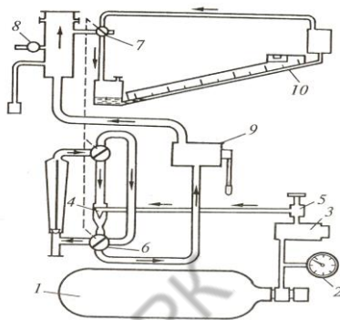
Рис. 128. Схема контрольного прибора УКП-5
