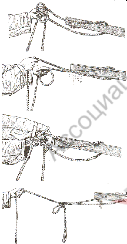
Рис.211. Закрепление спасательной бечевы (первый способ)
