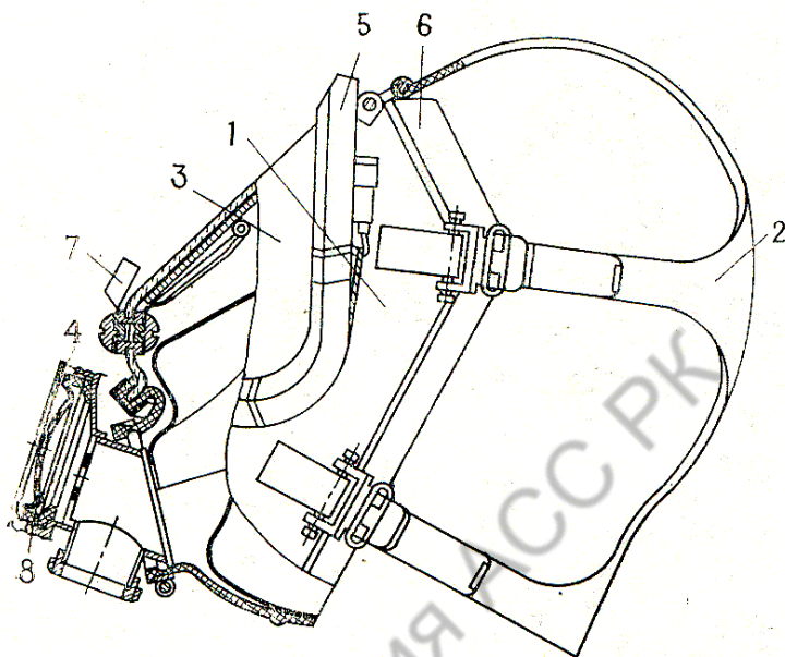
Рис. 26. Панорамная маска МПП
