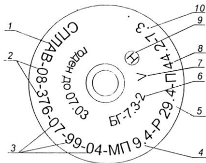
Рис. 19. Маркировка стального баллона баллона ГНПП «СПЛАВ»
