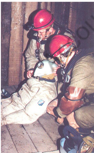
Рис.189. Включение пострадавшего в резервный респиратор
