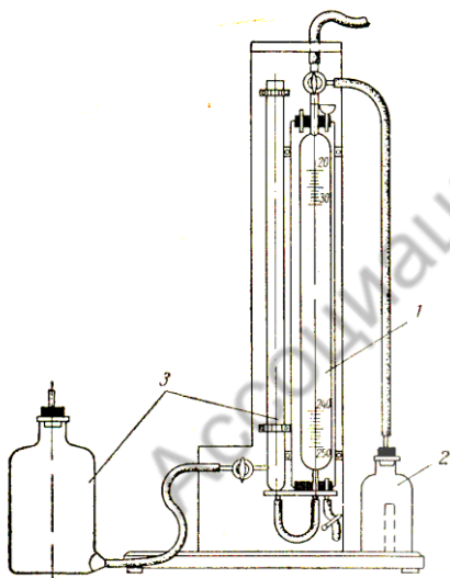
Рис.168. Прибор «Кальциметр» для определения содержания \text{CO}_2 в ХП-И объемным методом
