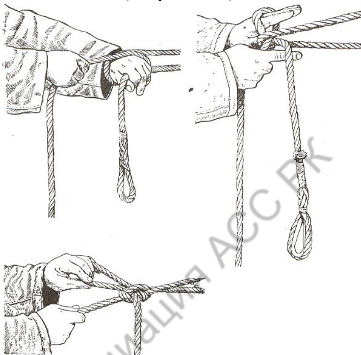
Рис.212. Закрепление спасательной бечевы вторым способом
