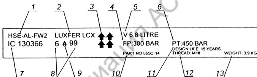
Рис. 21. Маркировка металлокомпозитного баллона Фирмы «LUXFER GAS CYLINDERS»
