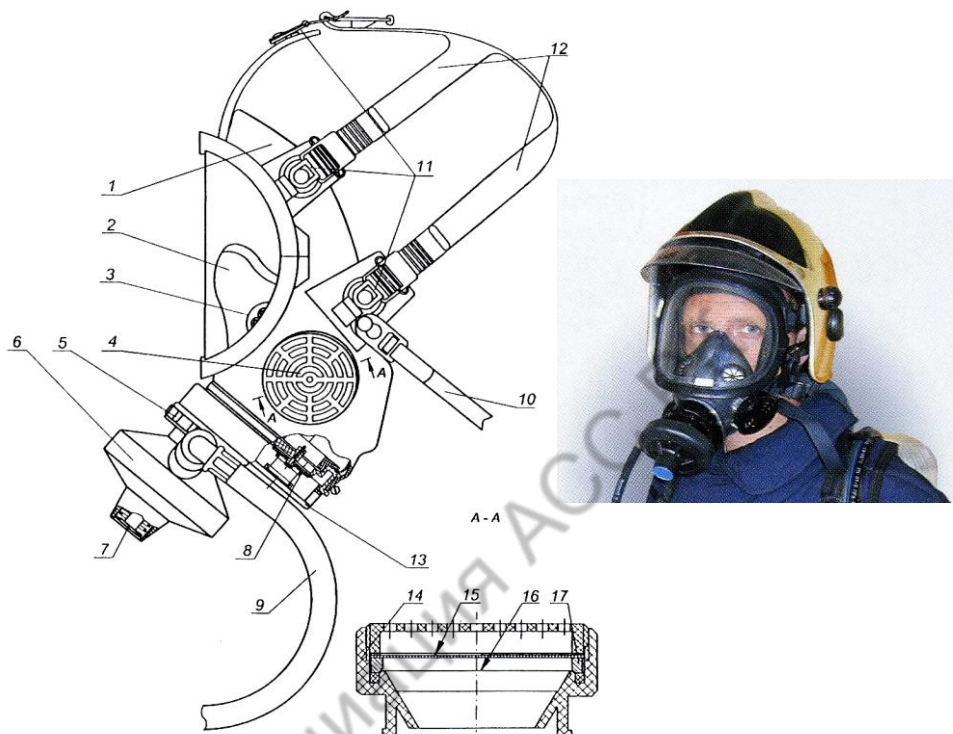
Рис. 28. Маска ПМ-2000 с легочным автоматом (вариант 1)
