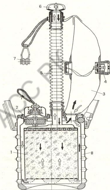
Рис. 14. Схема устройства ШСС-1
