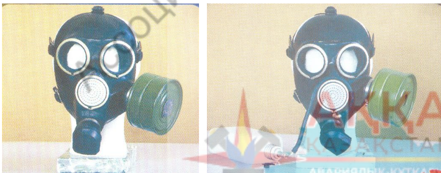
Рис.6. Гражданские противогазы: ГП-7 и его модификация ГП-7В
