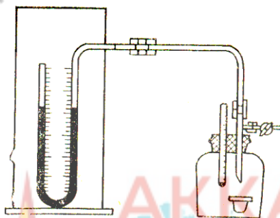
Рис.169. Прибор для определения содержания \text{CO}_2 в ХП-И манометрическим методом
