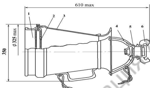
Рис. 118. Генератор пены средней кратности ГПС-600
